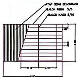
DETAIL PEKERJAAN ATAP Skala 1:50
